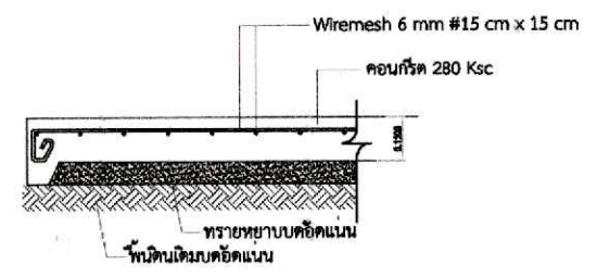
แบบขยายพื้นลานจอตกรถ
