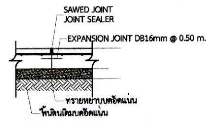
แบบขยายพื้น CONTRACTION JOINT
